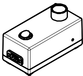
alimentation Speisegerät power unit 65 x 130 x 60 mm
